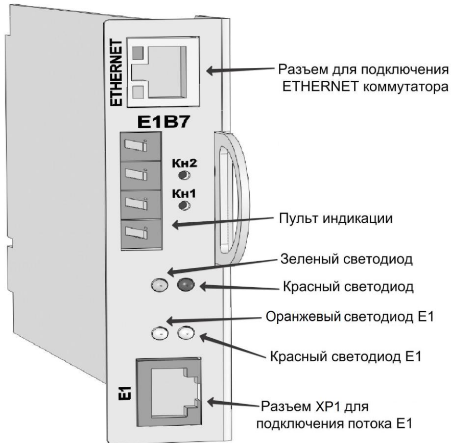
Рис. 15. Модуль E1B7
