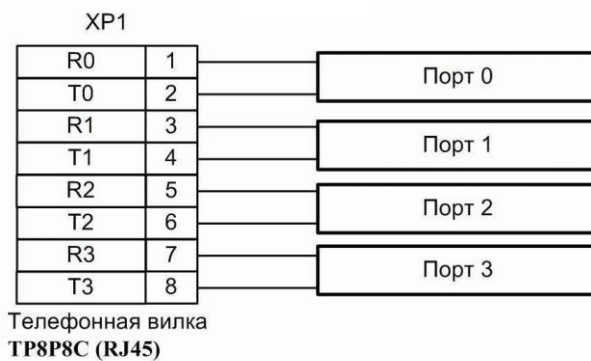
Рис. 30. Схема кабеля для подключения оконечных абонентских устройств к модулю DTB7-04
