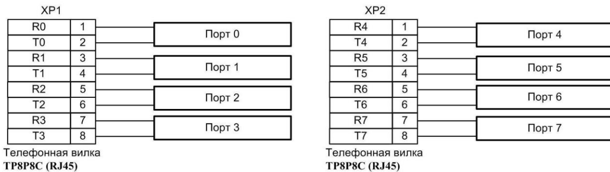
Рис. 4. Схема кабеля для подключения оконечных абонентских устройств
