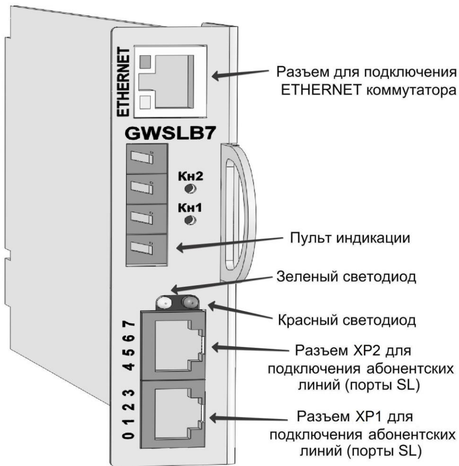
Рис. 19. Модуль GWSLB7
