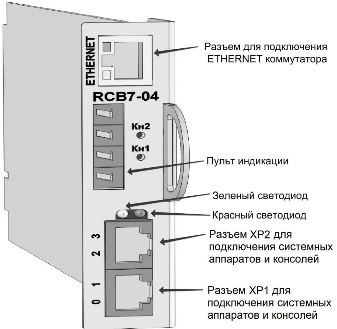
Рис. 12. Модуль RCB7-04
