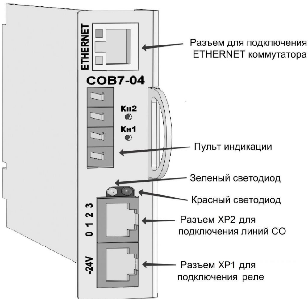
Рис. 5. Модуль COB7-04
